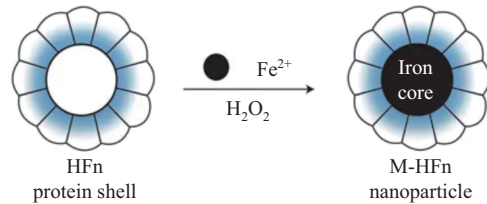
图6 人重链铁蛋白外壳内装载铁核 [20]
